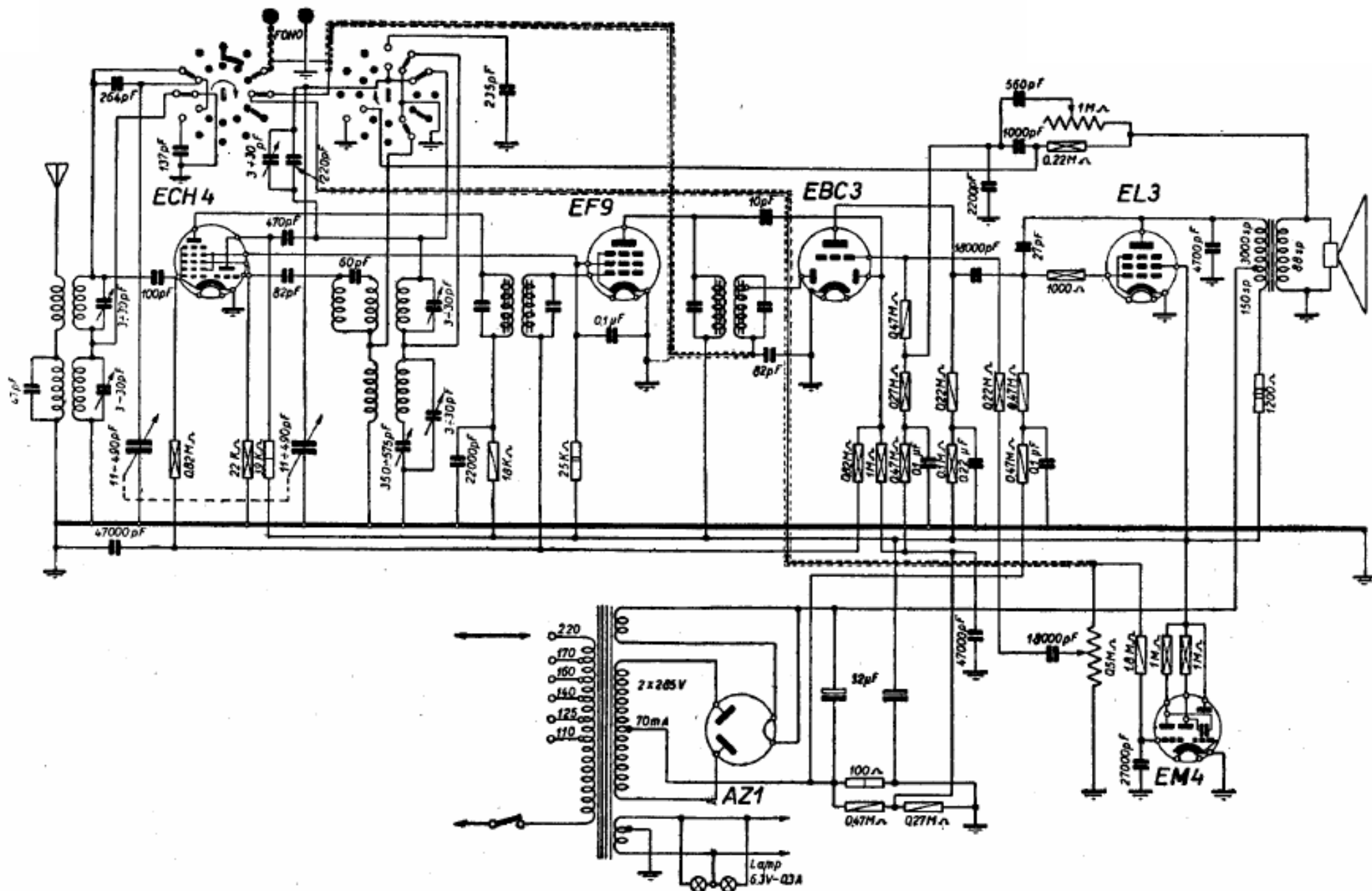
PHILIPS RADIO - Mod. BI 591 A - Ricevitore a gamme spostate. Media frequenza 468 kc. Massima tensione raddrizzata 290 V. Consumo 50 W. Potenza d'uscita 4 W.
